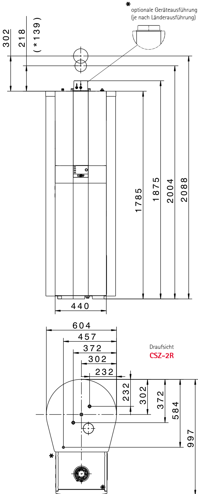
Vorderansicht CSZ-2R
